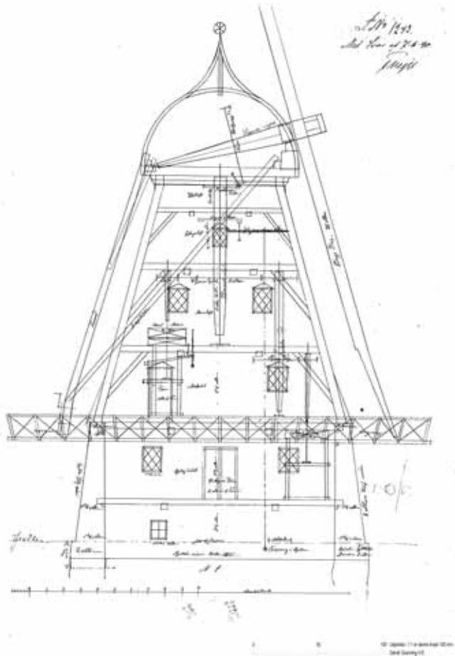
Snit af møllen. På vingen står 38 alen, hvilket svarer til knap 24 m. Tegning fra weblager.dk
