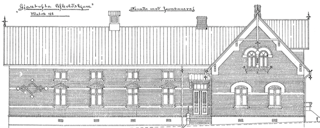
Adressen var tidligere Jernbanevej 24 og Brogårdsvej 24; nu er den Brogårdsvej 44. Facaden mod Brogårdsvej. Tegning weblager.dk
