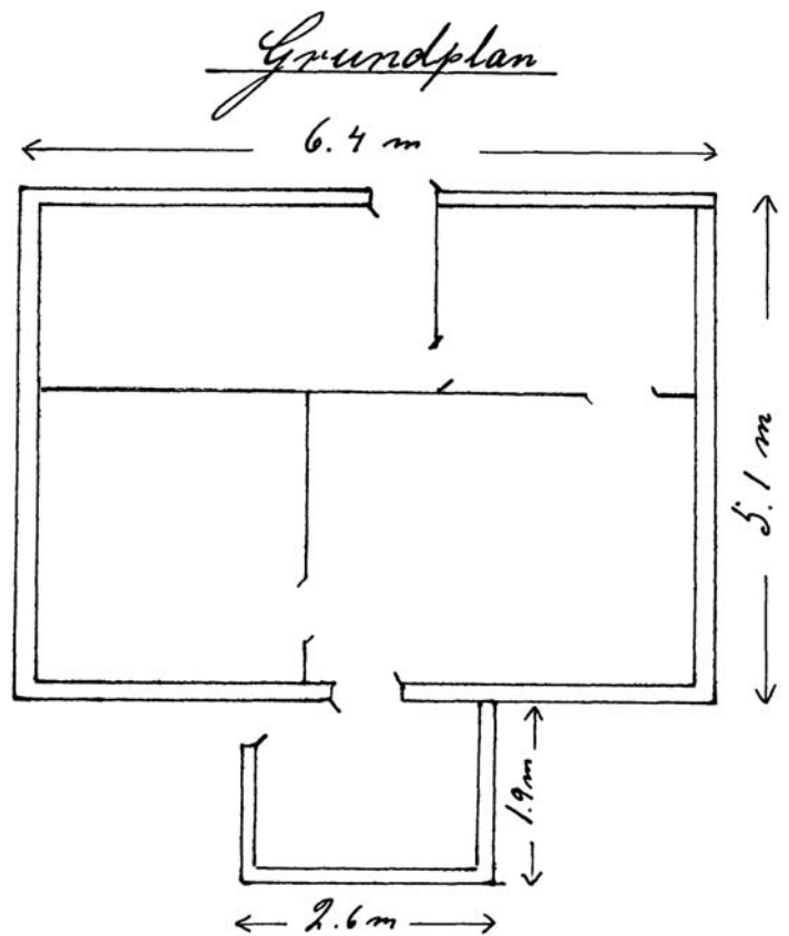
Træhusets grundplan. Kilde weblager.dk
